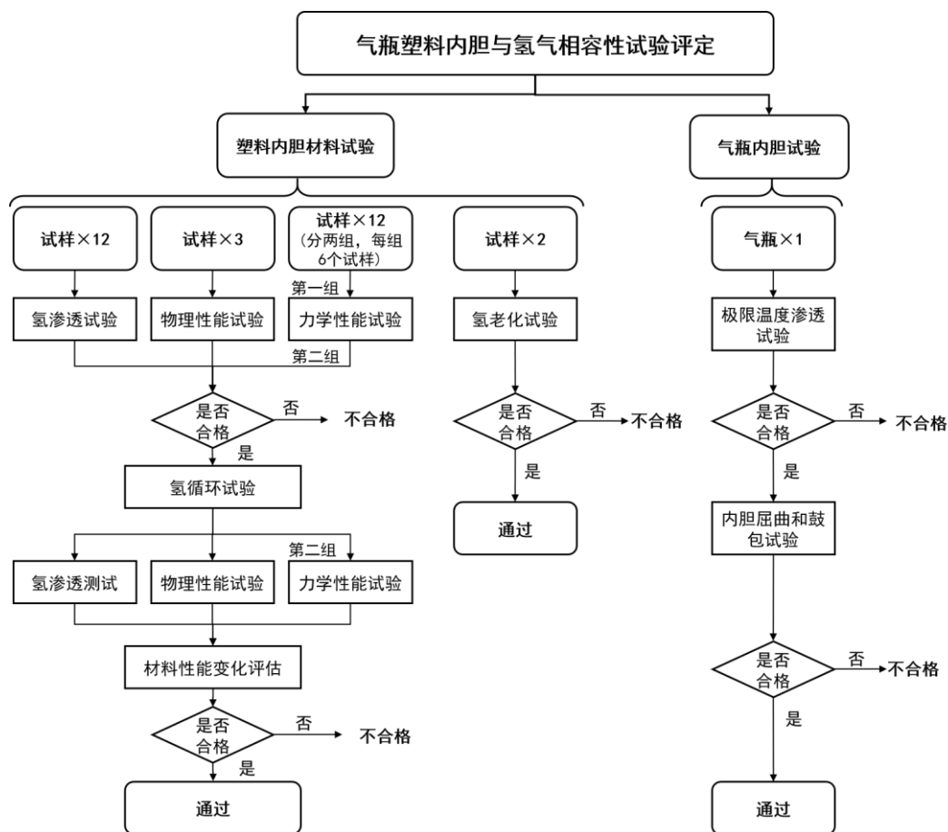
图A.1 气瓶塑料内胆与氢气相容性试验评定程序
