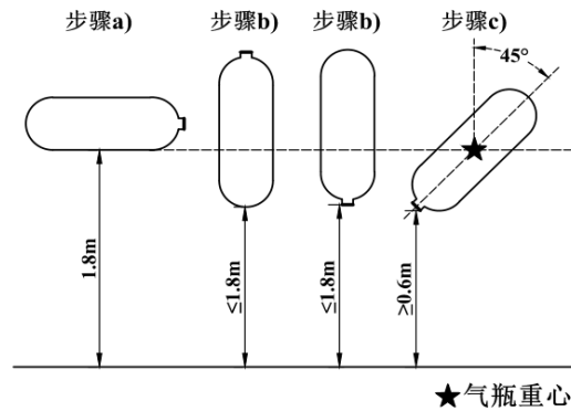
图6 跌落方向
