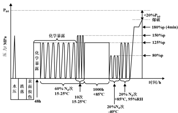
图7 耐久性试验
