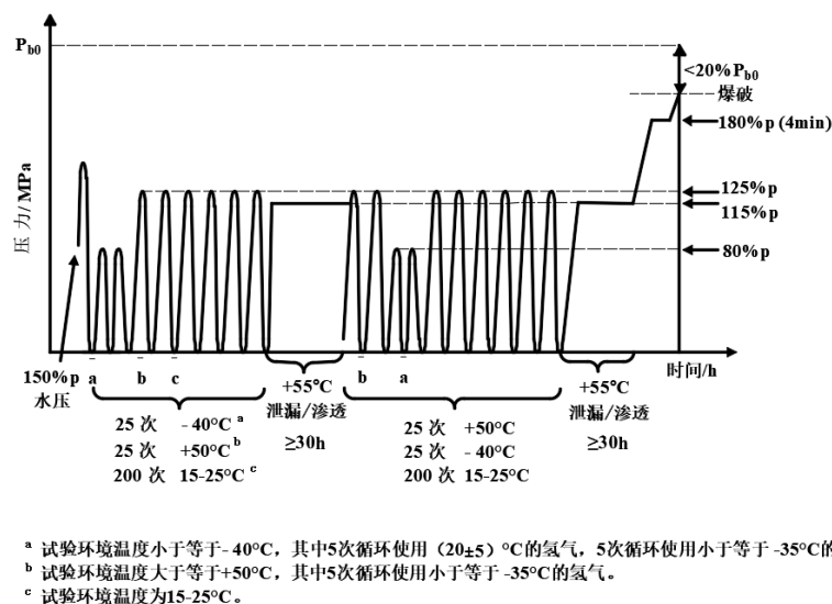
图 8 使用性能试验图示
